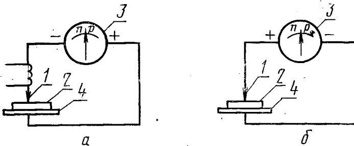
1 — зонд; 2 — образец; 3 — нуль-индикатор; 4 — металлическая пластинка
